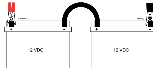
Esquema de ligação para duas baterias em série.
