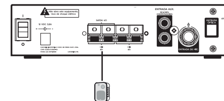
LIGAÇÃO 2 LIGUE 1 CAIXA DE 4Ω NA SAÍDA INDICADA
