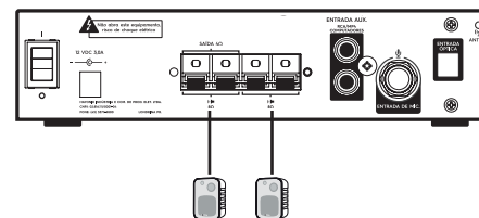
LIGAÇÃO 1 LIGUE ATÉ 2 CAIXAS DE 8Ω (1 POR CANAL)
